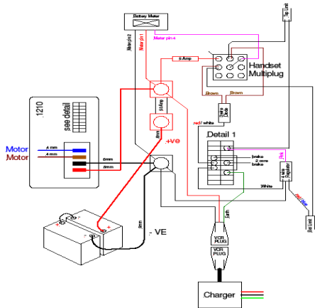
13. DIAGRAMA DE CONEXIONES ELÉCTRICAS PARA UNIDAD DE ACCIONAMIENTO ÚNICO
